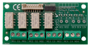
004666 UNii uitgang expansieprint 4 Relais Max. 1x per centrale of I/O
