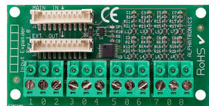
004664 UNii ingang expansieprint Max. 3x per centrale of I/O
