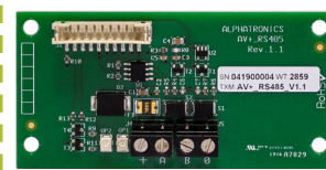
004663 UNii RS-485 expansie module
